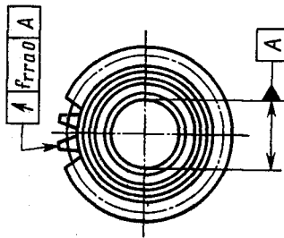
8. Отклонение диаметра окружности вершин зубьев f_{аа0}
