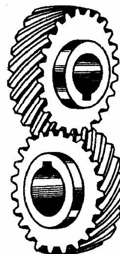
Рис. 7.3. Винтовая зубчатая передача
