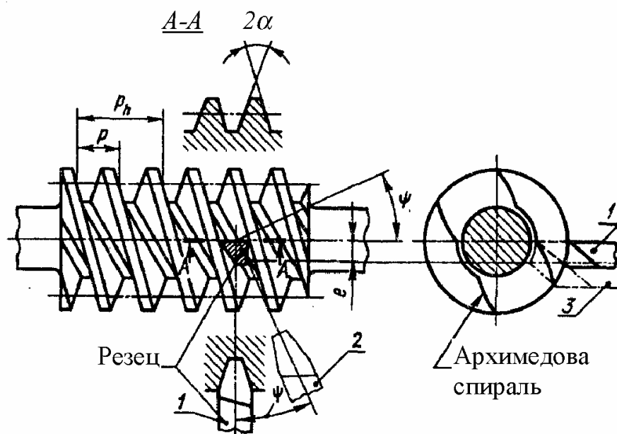
Рис. 11.4. Схема установки инструмента при нарезании червяка
