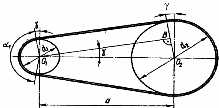
Рис. 13.2. Геометрические параметры ременной передачи
