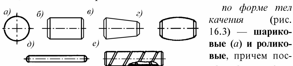
Рис. 16.3. Тела качения подшипников
