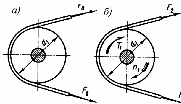
Рис. 13.3. Силы в ветвях ремня
