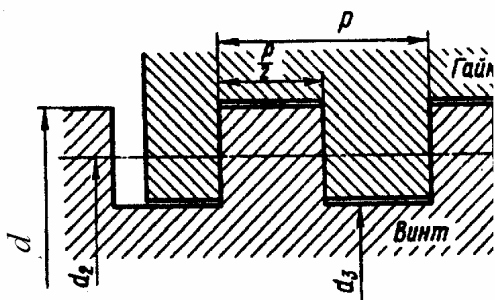
Рис 3.7. Прямоугольная резьба
