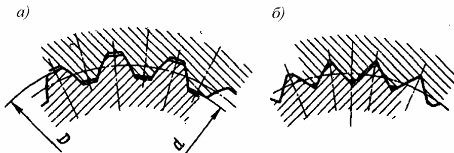
Рис 5.2. Эвольвентное ( а ) и треугольное ( б ) шлицевые соединения
