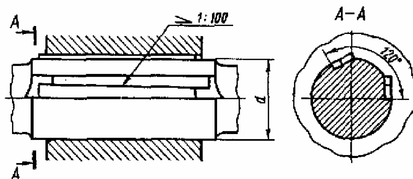
Рис 4. 4. Соединение тангенциальными шпонками
