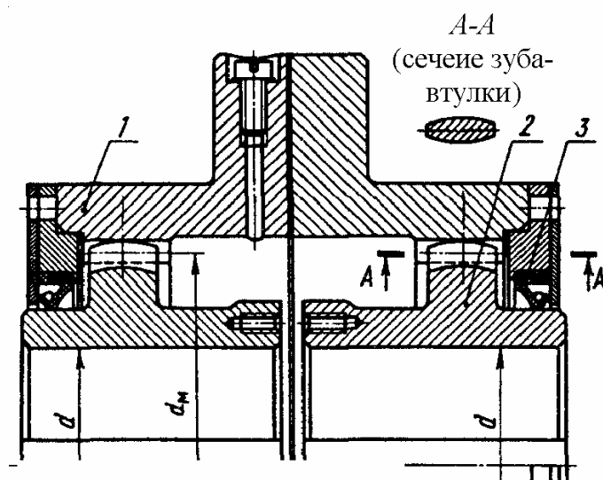
Рис. 17.4. Зубчатая муфта:
