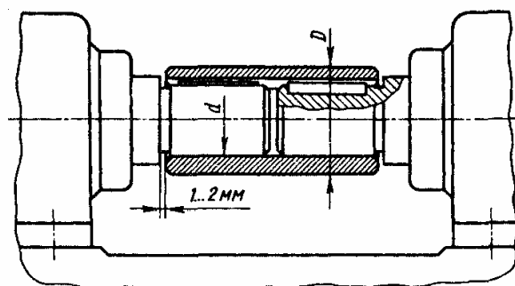
Рис. 17.1. Втулочная муфта
