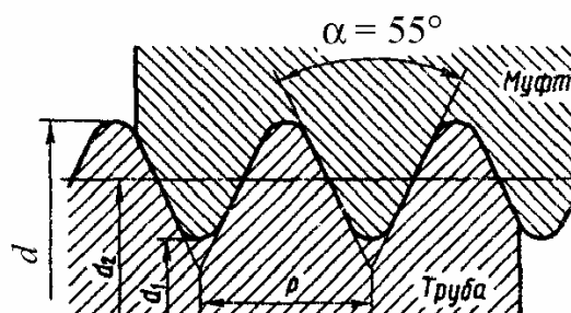
Рис. 3.4 Трубная резьба
