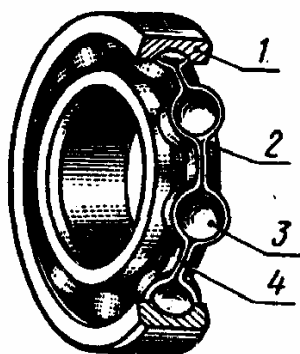
Рис. 16.1. Шариковый радиальный однорядный подшипник
