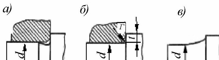
Рис. 15.4. Переходные участки вала
