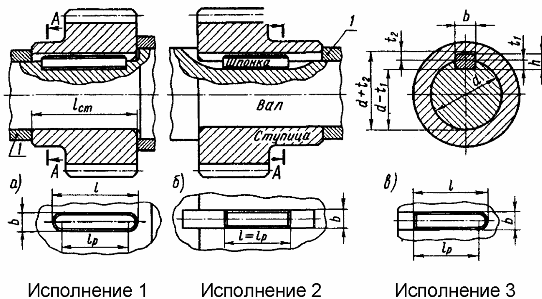
Рис. 4.1. Соединения призматическими шпонками
