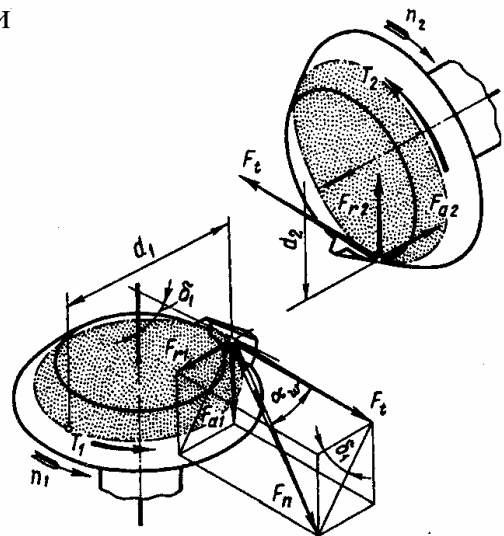
Рис. 10.4. Схема сил в конической прямозубой передаче (колеса условно раздвинуты)
