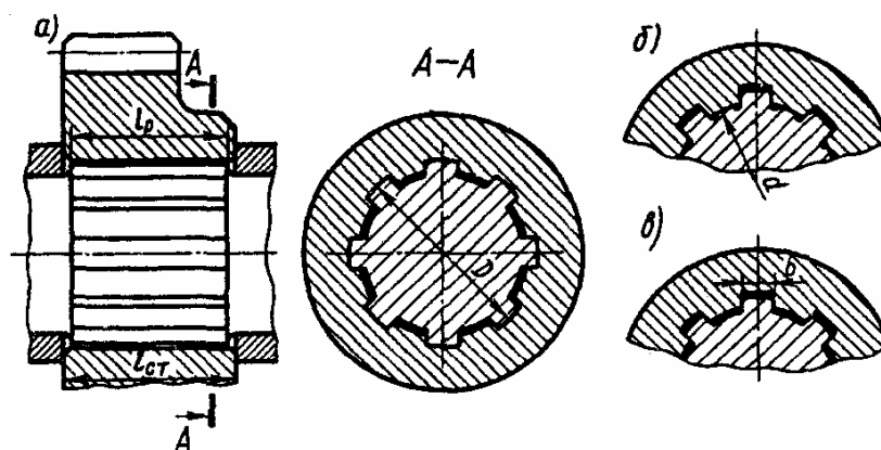
Рис 5.1. Прямоблочные шлицевые соединения
