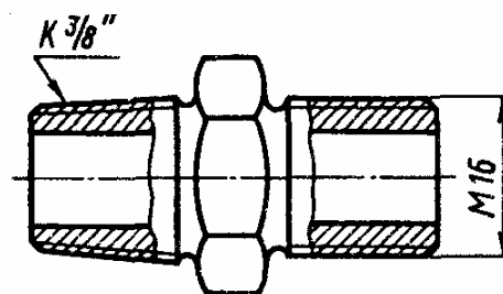
Рис.3.1. Пример конической и цилиндрической резьб
