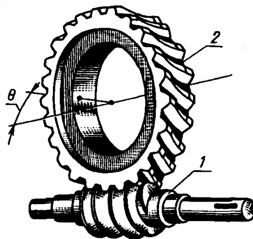
Рис. 11.1. Червячная передача:
