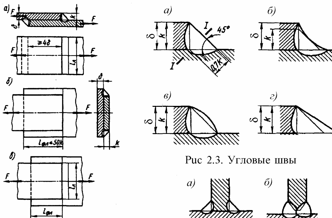
Рис. 2.2. Нахлесточные соединения угловыми швами
