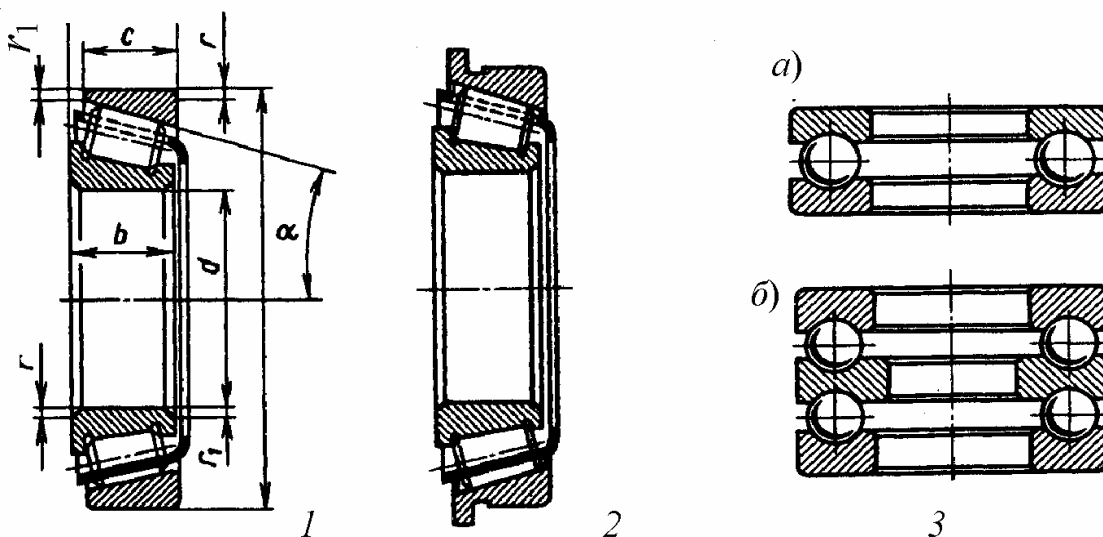
1 — Рис. 16.10. Роликовый конический подшипник
