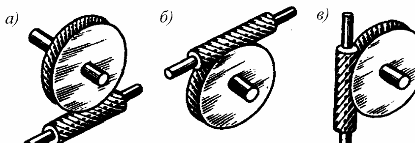
Рис. 11.3. Схемы расположения червяка относительно колеса
