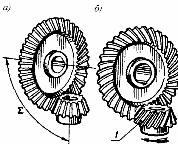
Рис. 7.2. Конические зубчатые передачи:
