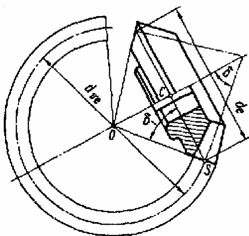
Рис. 10.3. Схема к определению эквивалентного числа зубьев
