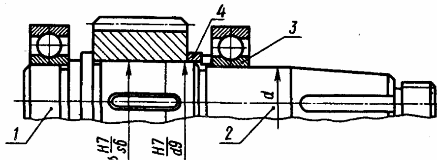
Рис. 15.2. Прямой ступенчатый вал:
