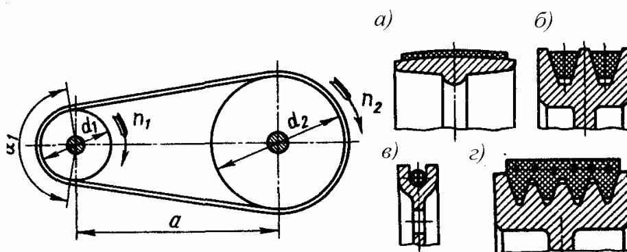
Рис. 13.1. Схема ременной передачи
