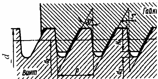
Рис 3.6. Упорная резьба
