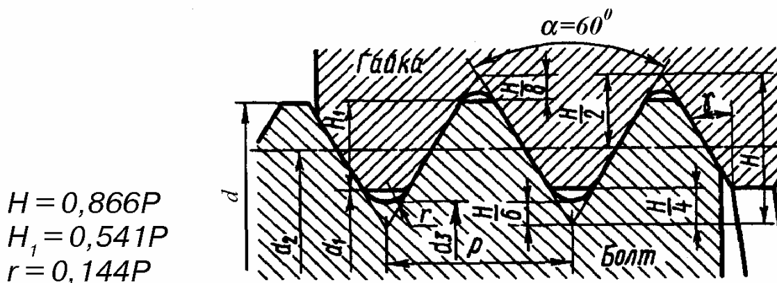
Рис. 3.3. Метрическая резьба
