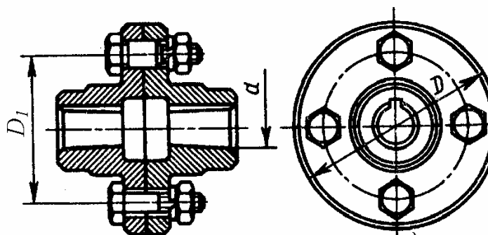
Рис. 17.2. Фланцевая муфта
