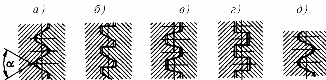
Рис. 3.2. Профили резьб
