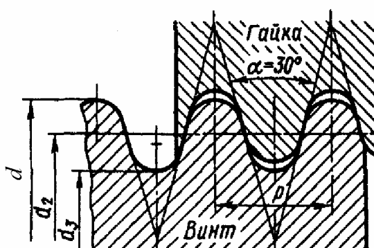
Рис 3.8. Круглая резьба
