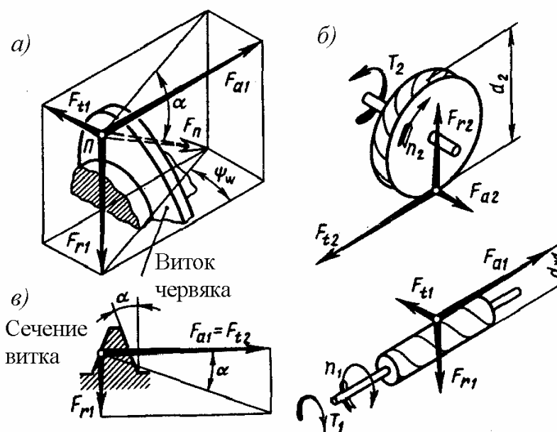
Рис. 11.8. Схема сил, действующих в червячном зацеплении
