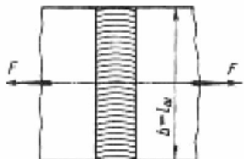
Рис. 2.5. Стыковые соединения
