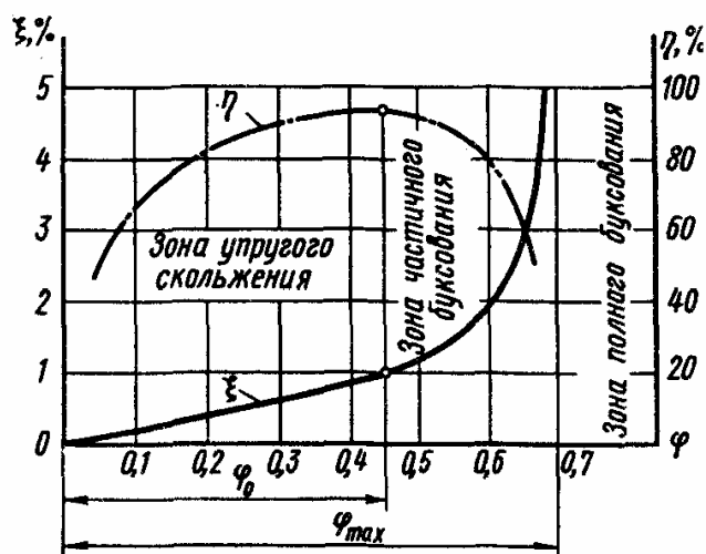
Рис. 13.7. Кривые скольжения и КПД
