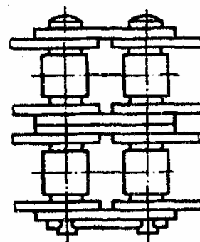
Рис. 14.3. Приводная втулочная двухрядная цепь
