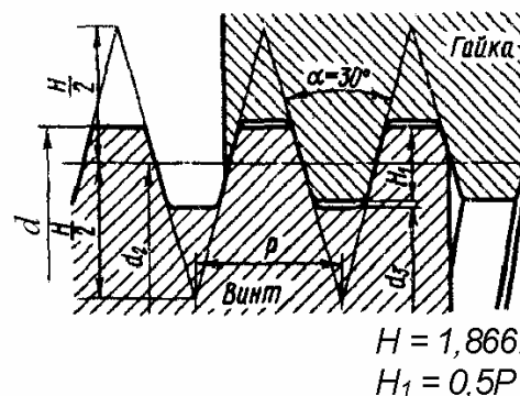
Рис. 3.5 Трапецеидальная резьба
