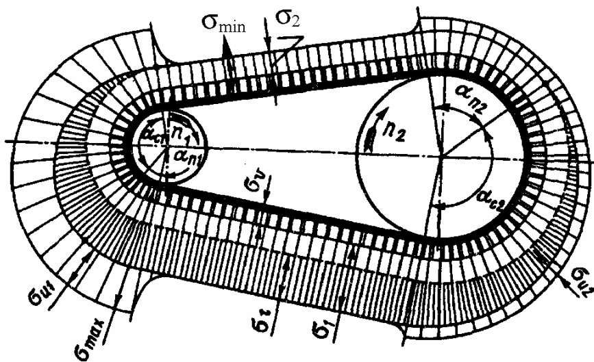
Рис. 13.6. Эпюра напряжений в ремне при работе передачи
