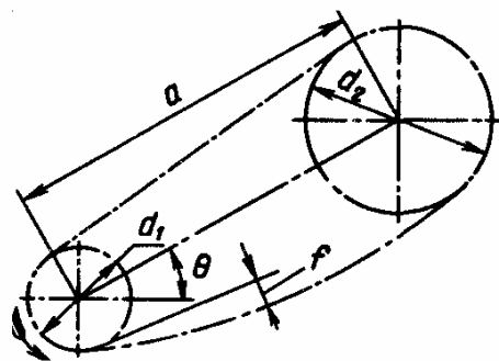
Рис. 14.7. Схема цепной передачи
