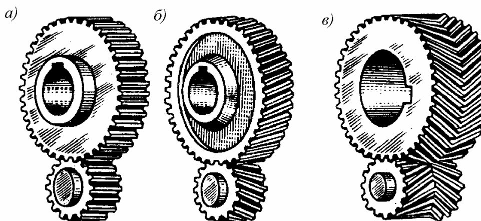
Рис. 7.1. Цилиндрические зубчатые передачи внешнего зацепления
