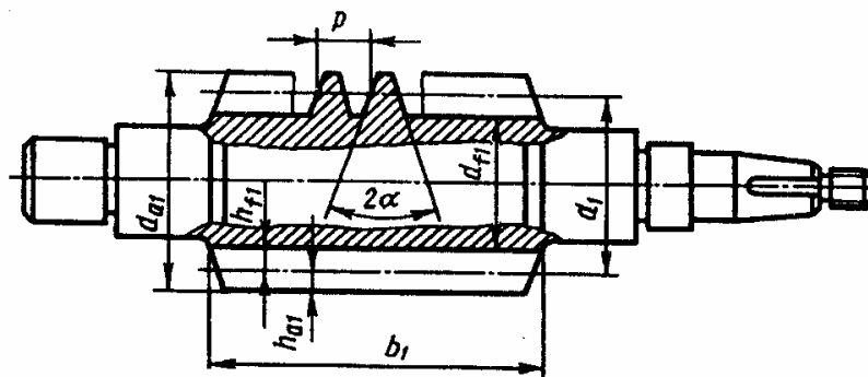
Рис. 11.5. Основные размеры цилиндрического червяка
