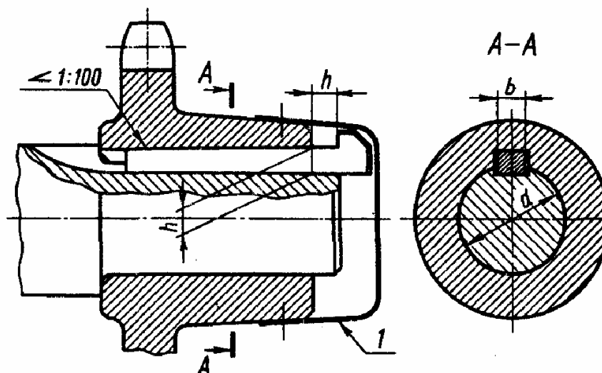
Рис. 4.3. Соединение клиновой шпонкой
