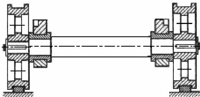
Рис. 15.1. Ось тележки
