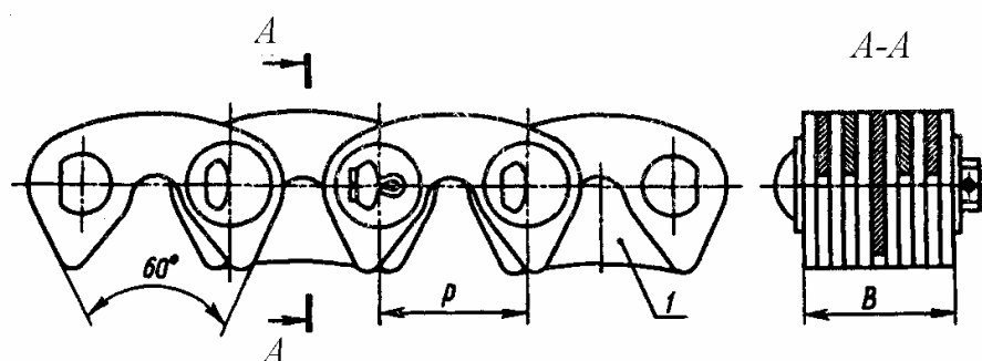
Рис. 14.4. Приводная зубчатая цепь
