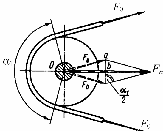
Рис. 13.4. К определению нагрузки на валы ременной передачи
