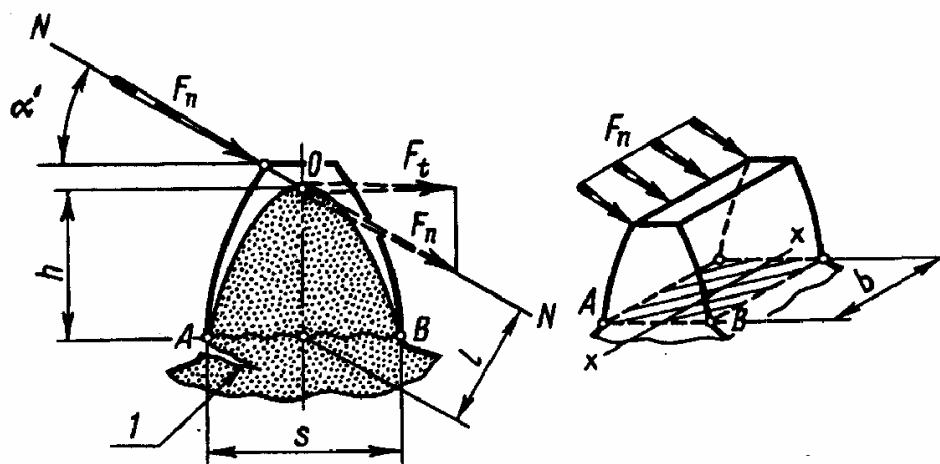
Рис 8.3, а. Схема к расчету зубьев на изгиб:
