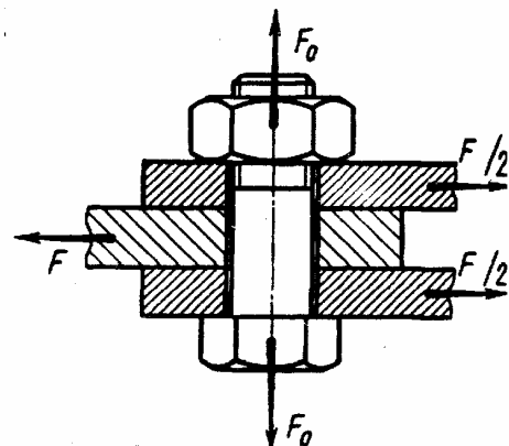
Рис. 3.10. Схема для расчета болтового соединения, нагруженного сдвигающей силой F
