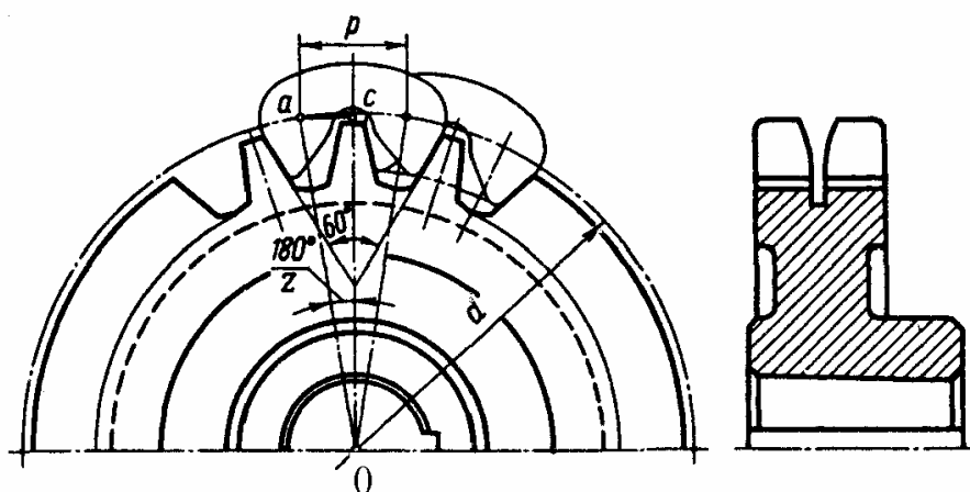
Рис. 14.6. Звездочка зубчатой цепи
