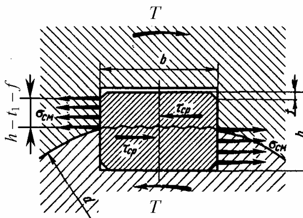
Рис 4.5. Расчетная схема соединения призматической шпонкой
