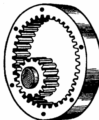
Рис. 7.5. Цилиндрическая прямозубая передача внутреннего зацепления
