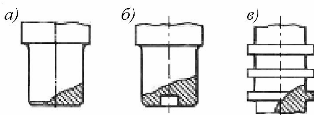
Рис. 15.3. Пяты
