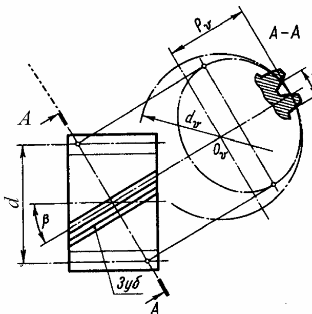
Рис. 9.2. Схема для определения z_v косозубого колеса
