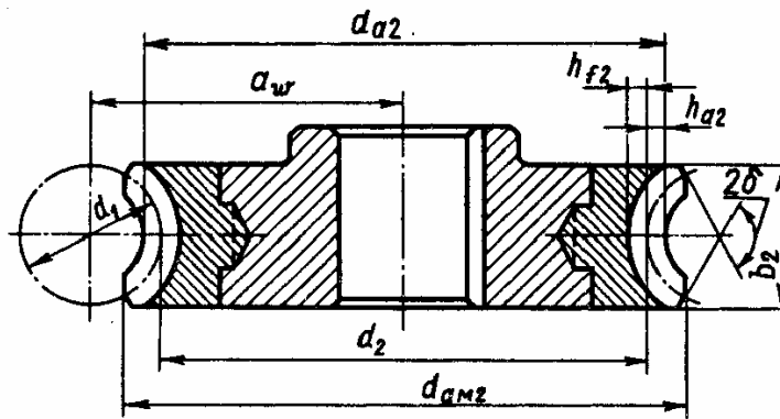
Рис. 11.7. Основные размеры венца червячного колеса
