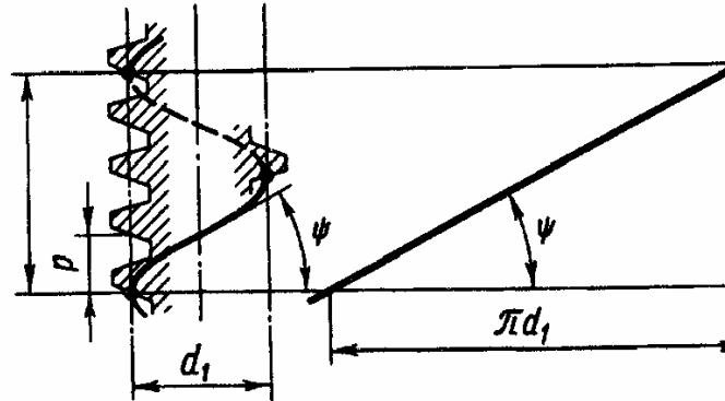
Рис. 11.6. Схема определения делительного угла подъема линии витка
