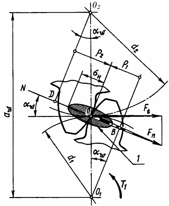
Рис. 8.2. Схема к расчету зубьев на контактную прочность: I — эпюра контактных напряжений
