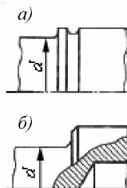
Рис. 15.5. Способы повышения уставной прочности валов
