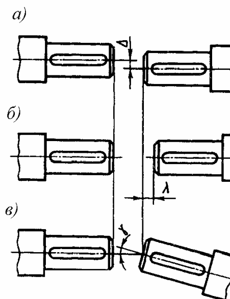
Рис. 17.3. Погрешности расположения валов:
